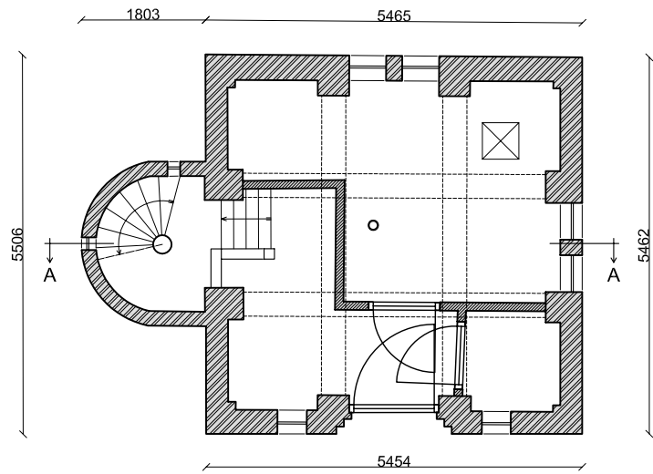
BEGANEGROND
