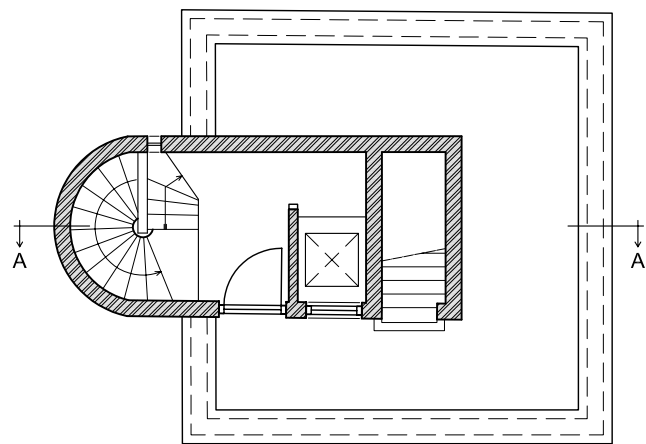
4E VERDIEPING
