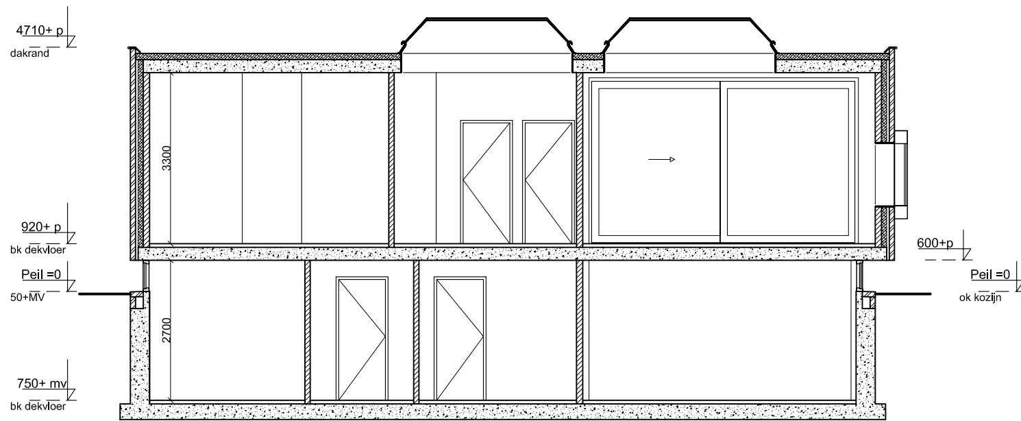
DOORSNEDE A-A
