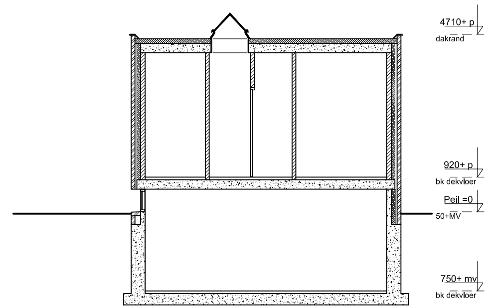
DOORSNEDE B-B
