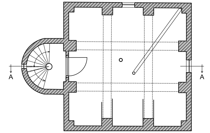
2E VERDIEPING
