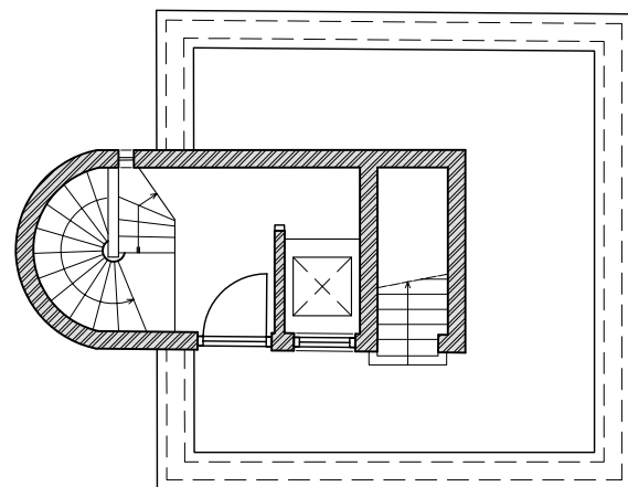
4E VERDIEPING
